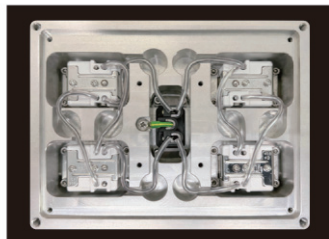
SBT-4X4 内部構造
